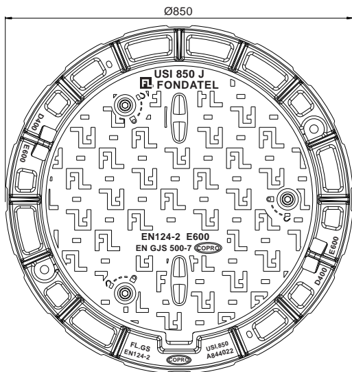
Vergrendelen en ontgrendelen via zeskantbout
