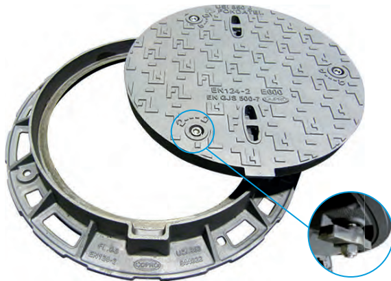
Vergrendelen en ontgrendelen via zeskantbout
