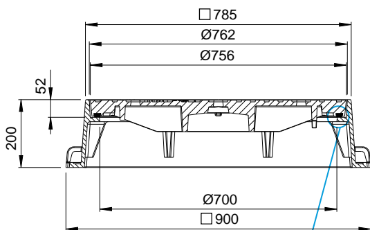
EPDM dichting
